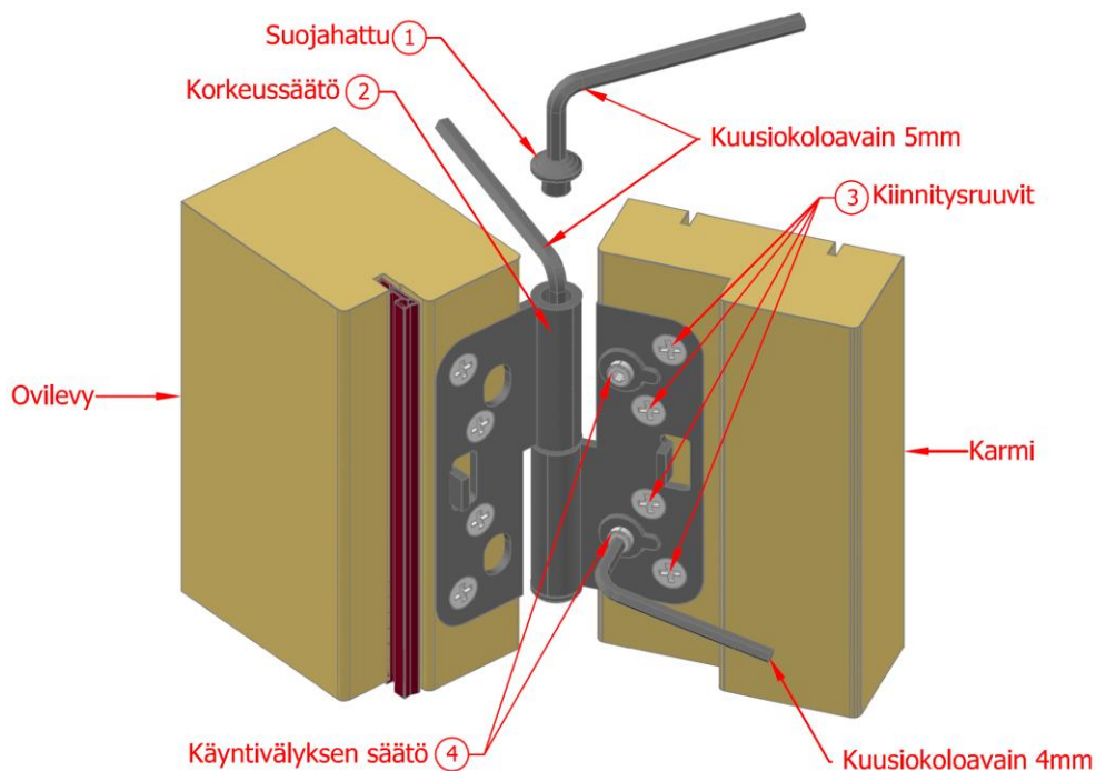
Kuva 3. Saranoiden säätäminen
