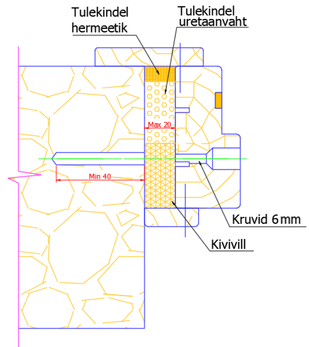
Joonis 2. Ukselengi ja tarindiava vaheline paigalduspiilu täidetakse kivivillaga ja tulekindla uretaanvahuga ning tihendatakse ruumi poolt tulekindla hermeetikuga
