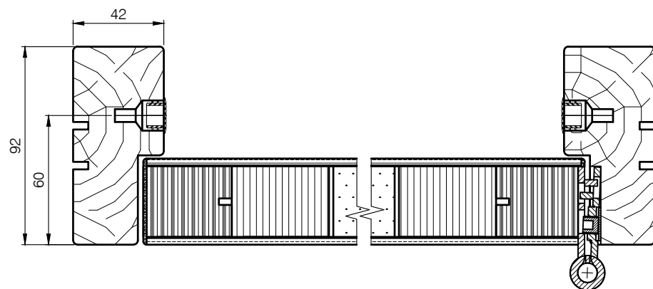
SSU NIISKUSKINDEL (leng põrandast -30 mm) Paigaldus.
