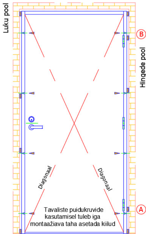
Joonis 1. Ukselengi fikseerimine tarindiavasse. Vältimaks lengide väändumist ja tihedamaks püstlengide ja ülapii ning ukseläve vahelisi pragusid, tuleb paariskiilud või tugiklotsid asetada ka ala- ja ülannurkadesse
