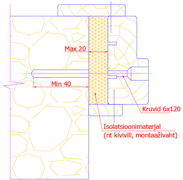
Joonis 2. Ukselengi ja tarindiava vaheline paigalduspilu täidetakse isolatsioonimaterjaliga (nt kivivill, klaasvill, montaaživaht). Vahu kasutamisel jälgige, et vahul oleks paisumiseks ruumi ja peale paisumist ei ulatuks vahu servad üle lengi ääre.
