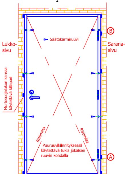
Kuva 1. Ovenkarmin kiinnitys rakenteen aukkoon. Karmien vääntymisen välttämiseksi pystykarmien ja yläpuun sekä kynnyksen rakojen tiivistämiseksi tulee parikiilat tai tukipalikat asettaa myös ala- ja ylänurkkiin
