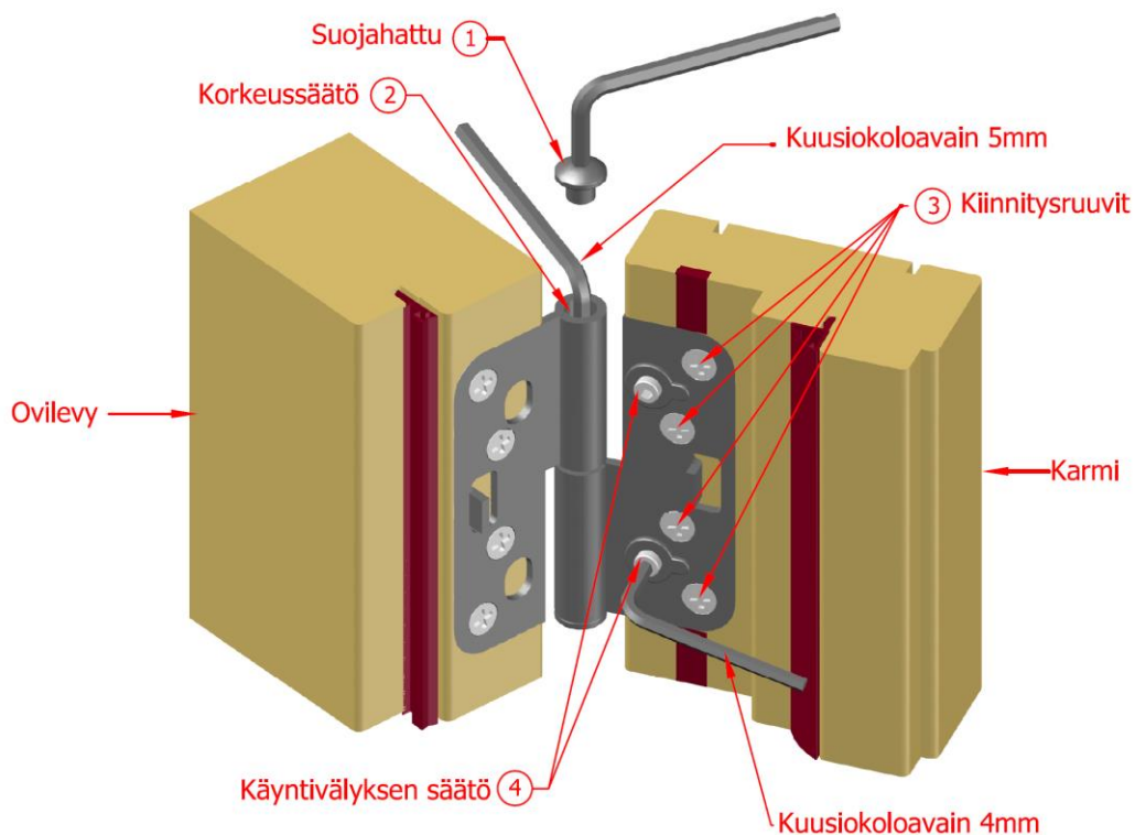
Kuva 3. Saranoiden säätäminen
