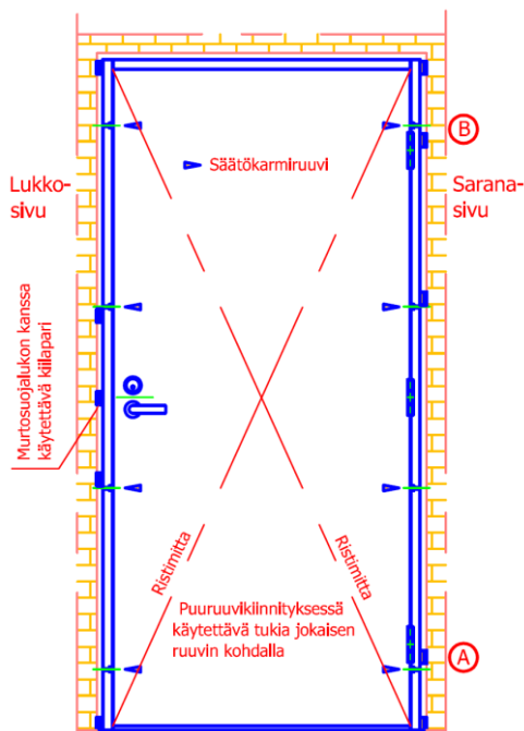
Kuva 1. Ovenkarmin kiinnitys rakenteen aukkoon. Karmien vääntymisen välttämiseksi pystykarmien ja yläpuun sekä kynnyksen rakojen tiivistämiseksi tulee pariikiilat tai tukipalikat asettaa myös ala- ja ylänurkkiin
