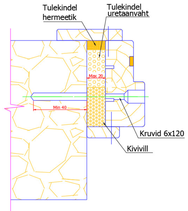
Joonis 2. Ukselengi ja tarindiava vaheline paigalduspilu täidetakse kivivilla ja tulekindla uretaanvahuga ning tihendatakse ruumi poolt tulekindla hermeetikuga
