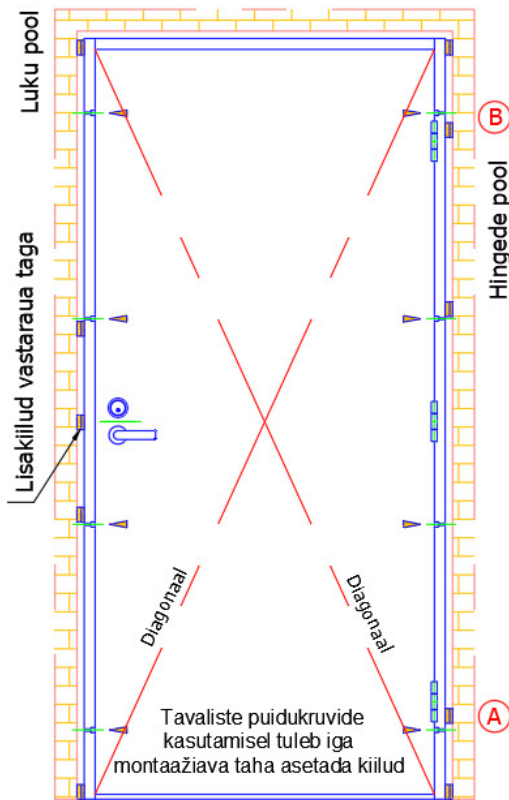
Joonis 1. Ukselengi fikseerimine tarindiavasse. Vältimaks lengide väändumist ja tihendamaks püstlengide ja ülapii ning ukselehe vahelisi pragusid, tuleb paariskiilud või tugiklotsid asetada ka ala- ja ülanurkadest
