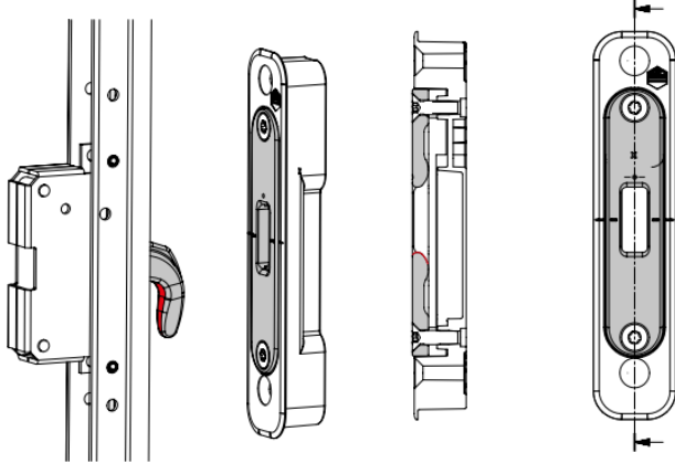
Maco Panoraman voitelupisteet
