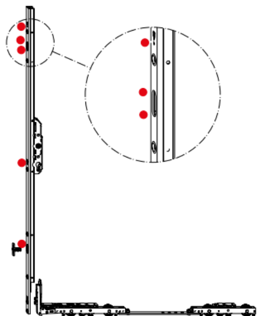
Roto Patio Lifen voitelupisteet
