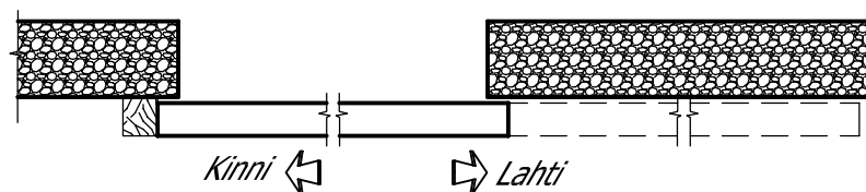
Paremakäeline lükanduks
